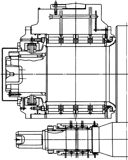
双推力圆锥滚子轴承的组装示例
