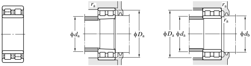
图例2-P (NNU型)
