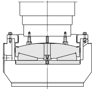
旋压用 推力圆锥滚子轴承的组装示例
